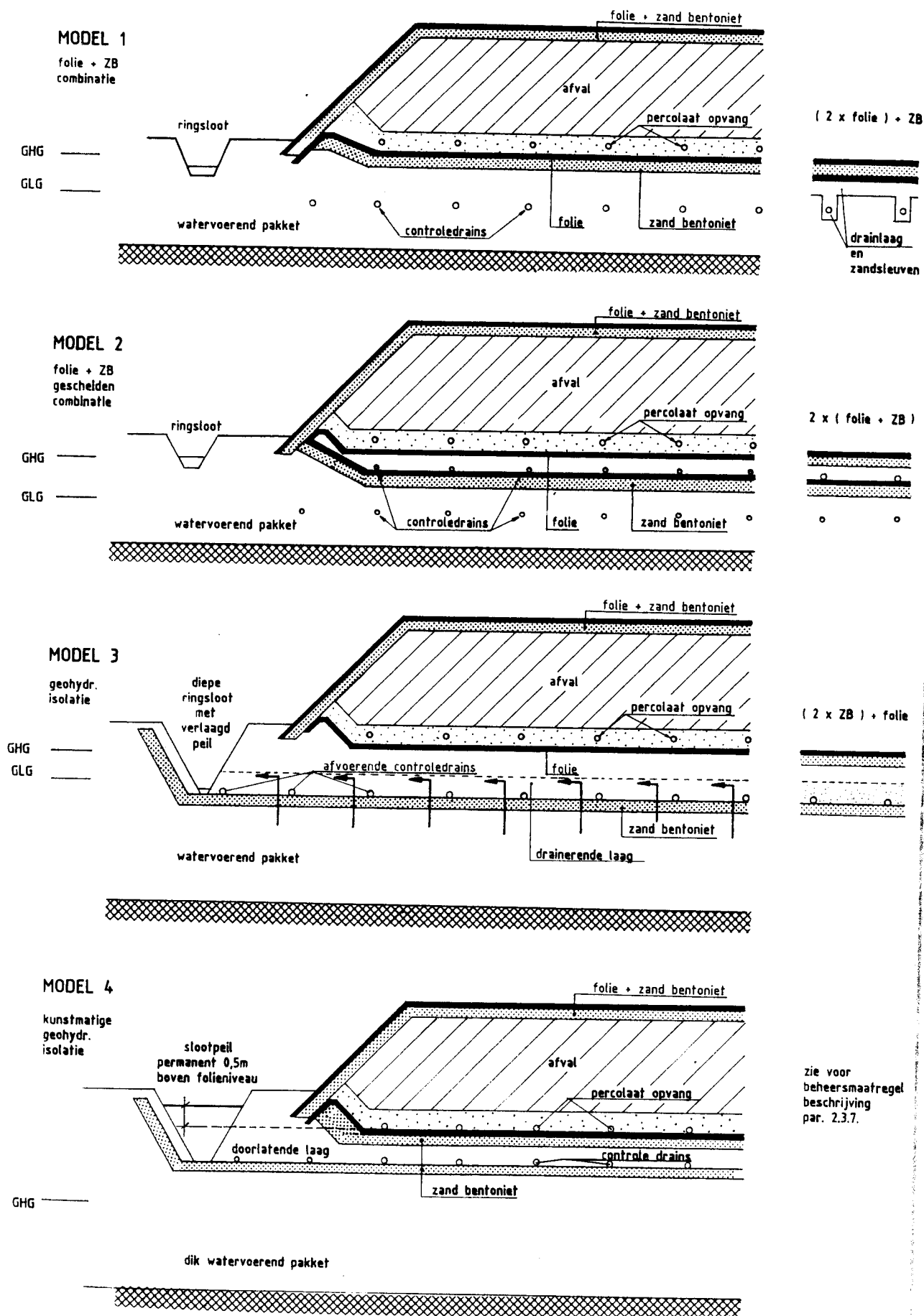
figuur 4 Onderafdichtingsconstructies
